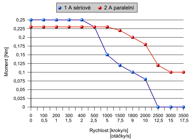
Momentová charakteristika motoru SL23-0704 s jednotkou CD20M a napájecím napětím 35 VDC
