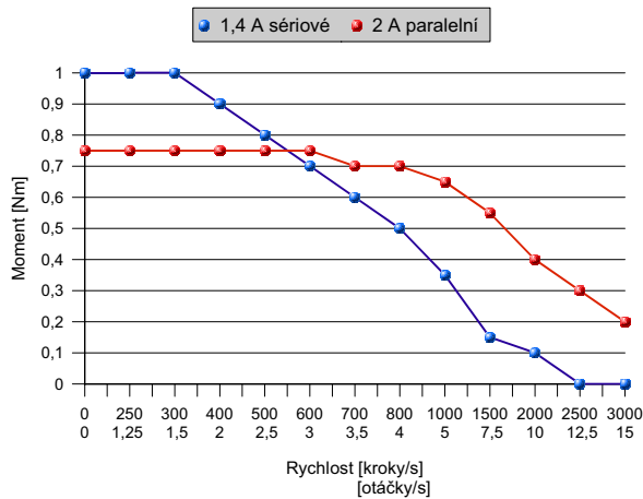
Momentová charakteristika motoru SL23-1012 s jednotkou CD20M a napájecím napětím 35 VDC
