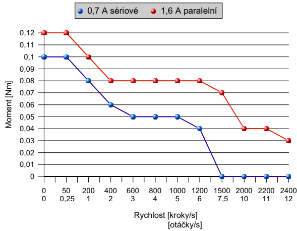
Momentová charakteristika motoru SL17-0601 s jednotkou CD20M a napájecím napětím 35 VDC
