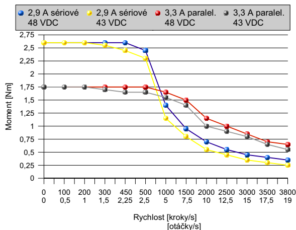
Momentová charakteristika motoru SL34-2530 s jednotkou CD30M a napájecím napětím 43 VDC a 48 VDC
