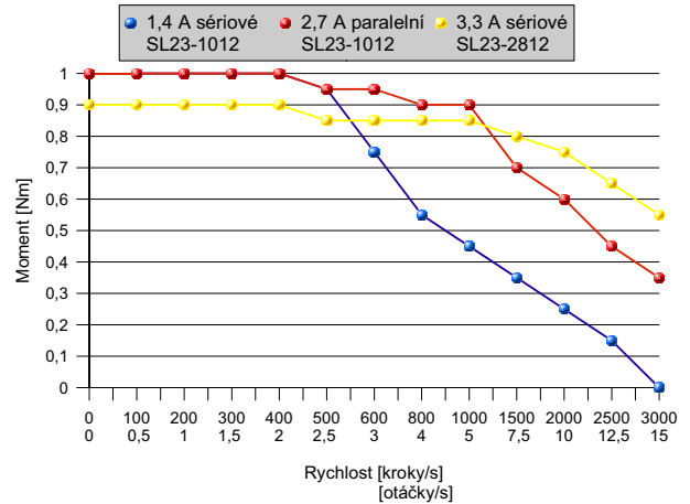
Momentová charakteristika motoru SL23-1012 (SL23-2812) s jednotkou CD30M a napájecím napětím 48 VDC
