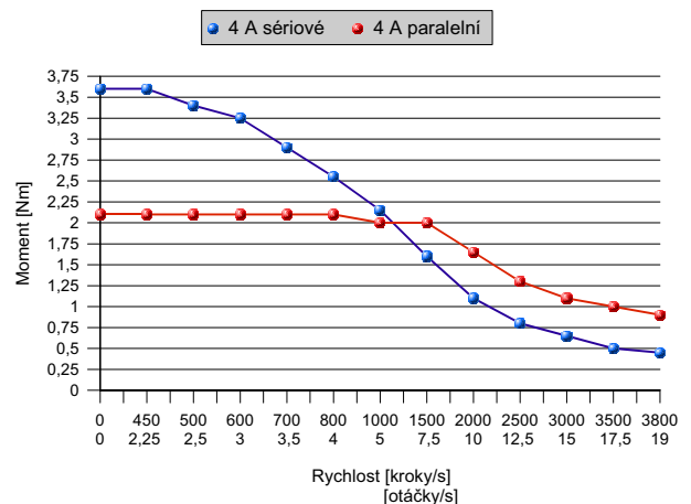
Momentová charakteristika motoru SL34-3550 s jednotkou CD40M a napájecím napětím 48 VDC
