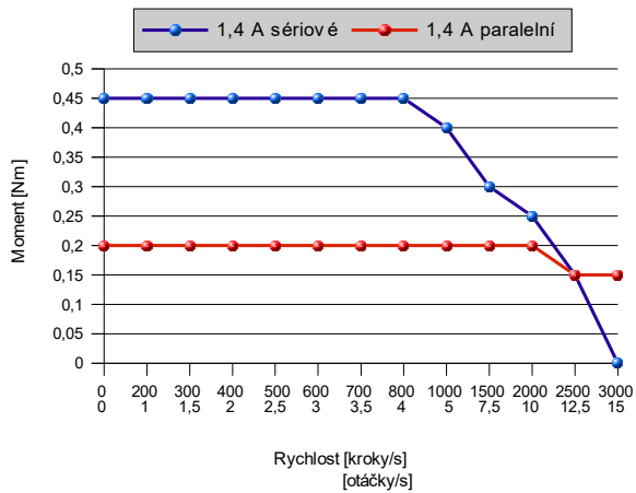
Momentová charakteristika motoru SM2317-0800 s jednotkou CD20M a napájecím napětím 35 VDC
