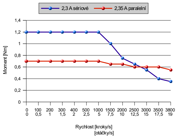
Momentová charakteristika motoru SM2321-1400 s jednotkami CD30x, CD30M a napájecím napětím 48 VDC
